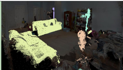
语义高斯
