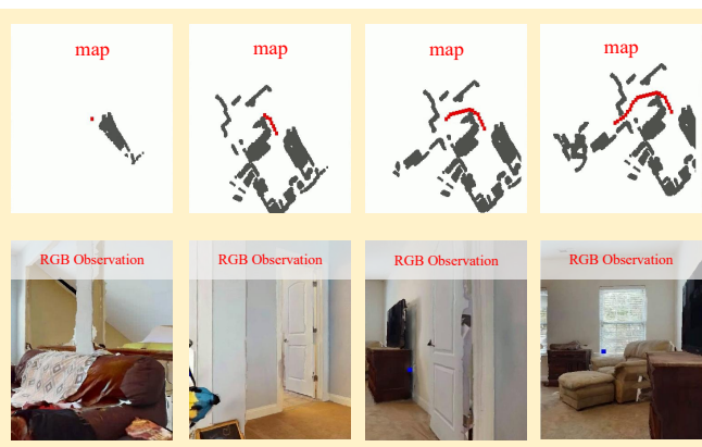
导航时间步
