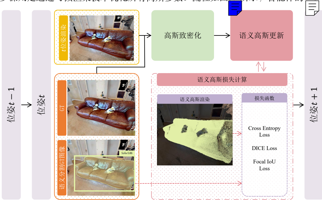
图 3.2 语义高斯渲染流程
