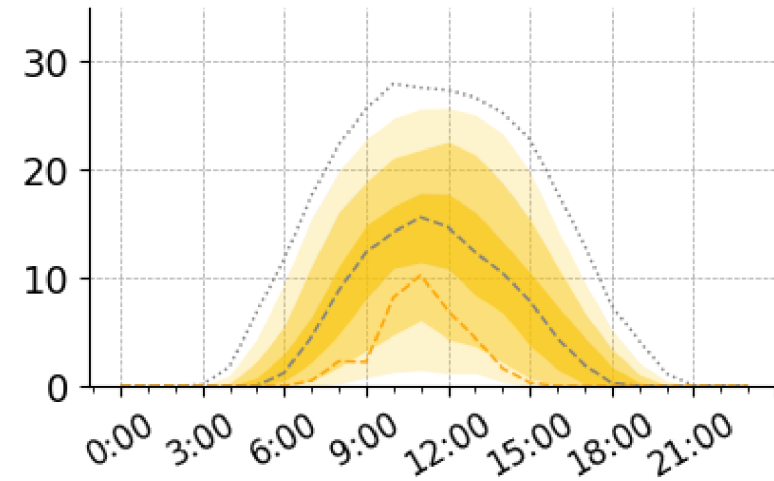
Inverter 2 (kW)
