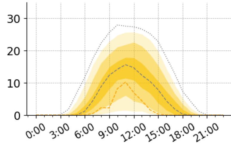
Inverter 2 (kW)
