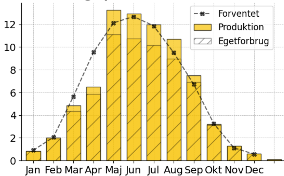
Månedlige produktionsværdier (MWh)
