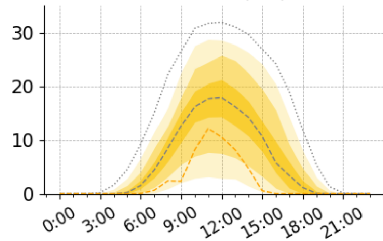
Inverter 2 (kW)
