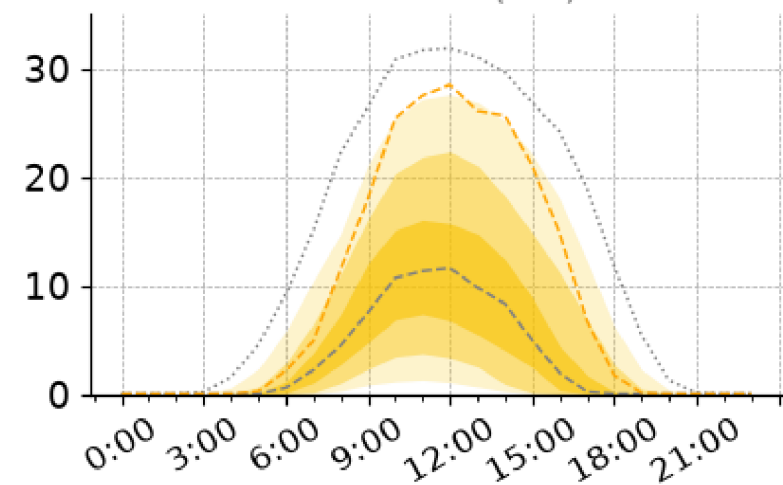
Inverter 2 (kW)
