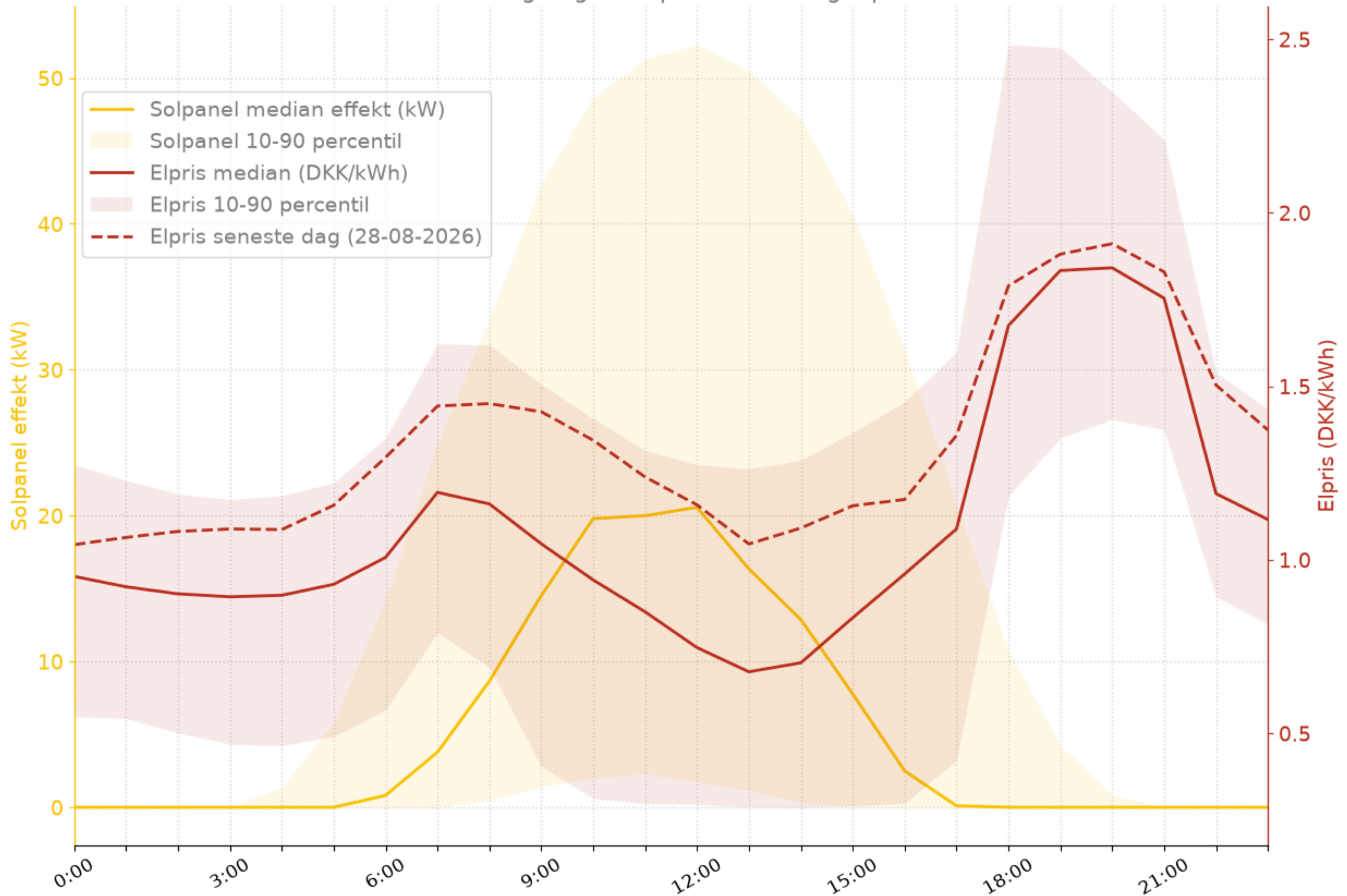
Sammenligning af solpanel effekt og elpriser
