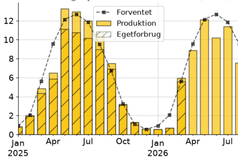
Daglig produktion (kWh)
