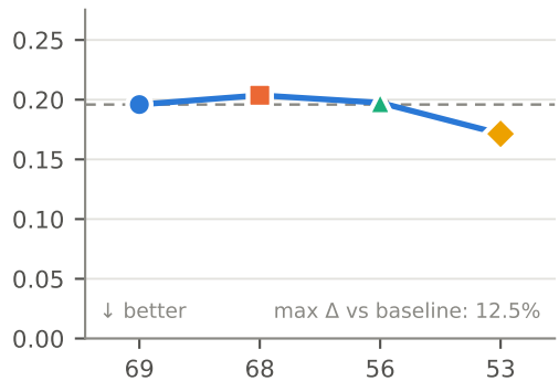
|e_{v_x}| [m/s]
