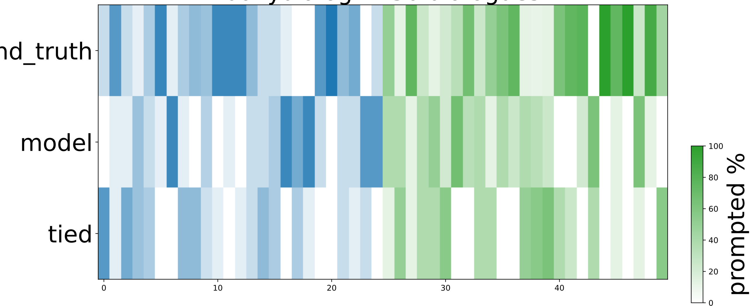
multiwoz — 50 dialogues
