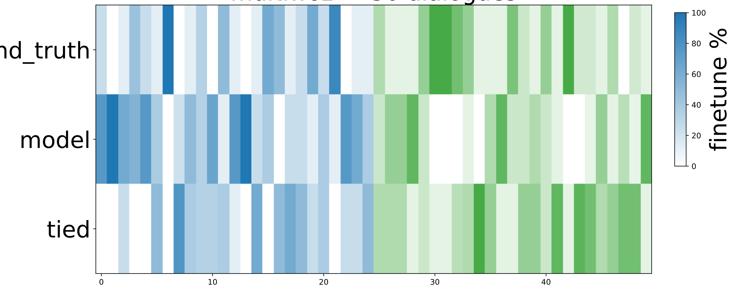
multiwoz — 50 dialogues
