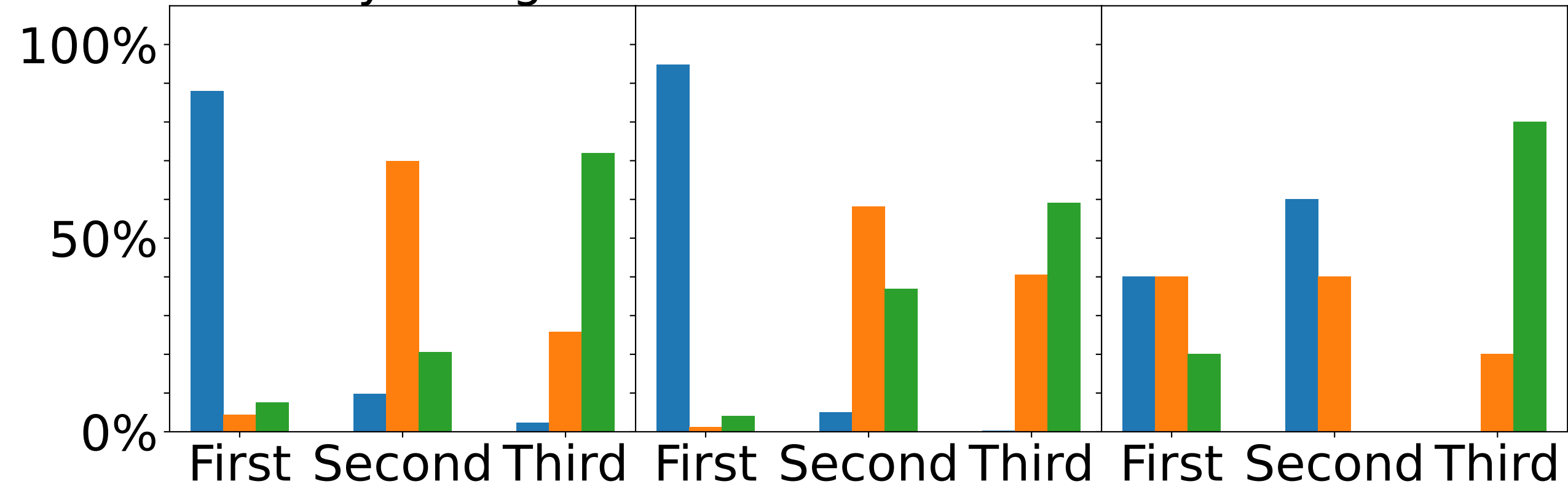
MultiWOZ
