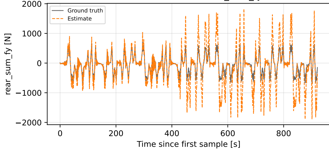
Baseline-NN-MSE - rear_sum_fy
