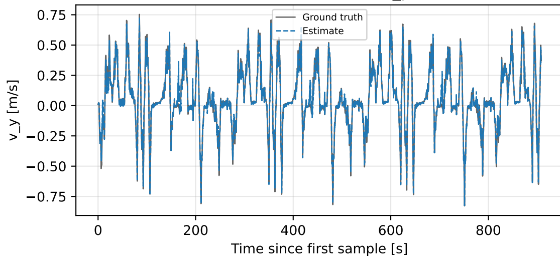
Baseline-NN-MSE - v_y
