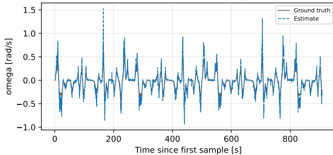
Baseline-NN-MSE - \omega
