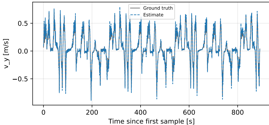
Baseline-NN-MSE - v_y
