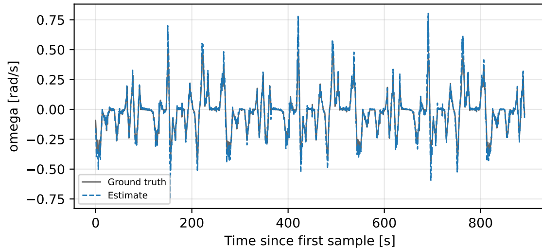
Baseline-NN-MSE - \omega
