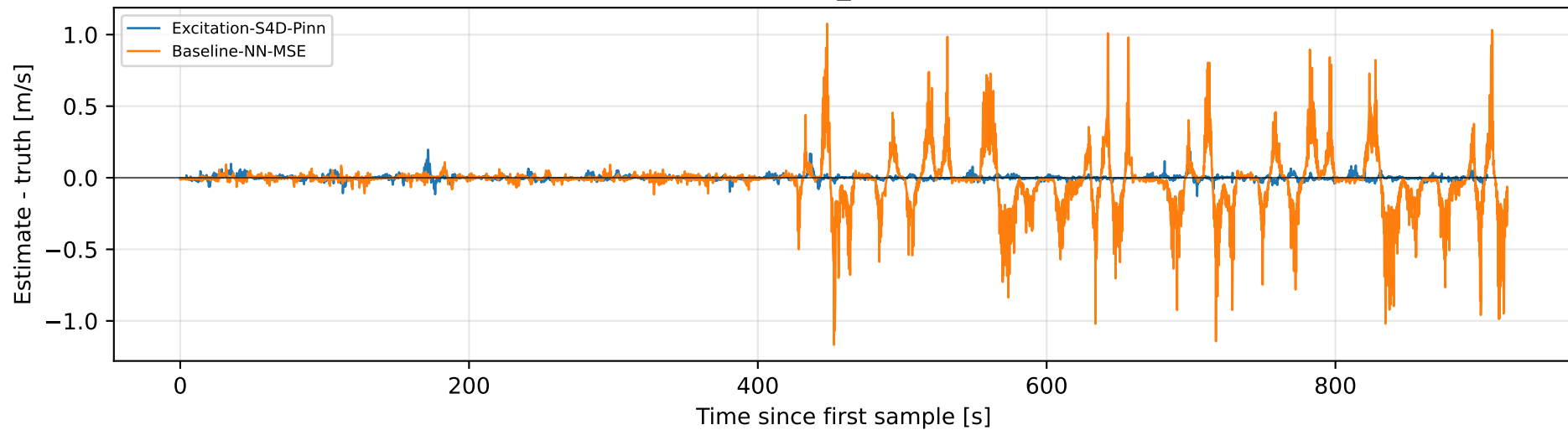
State estimation error per scenario
