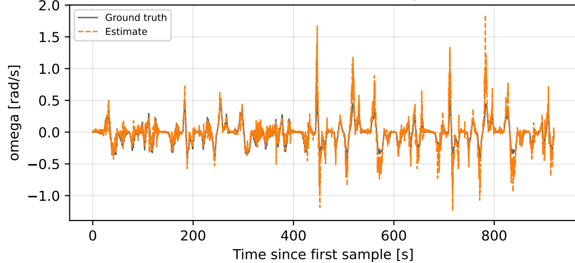
Baseline-NN-MSE - \omega
