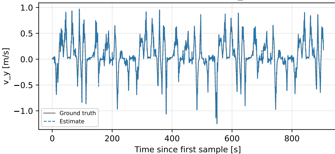
Baseline-NN-MSE - v_y
