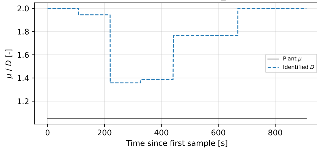
Baseline-NN-MSE - rear_mu
