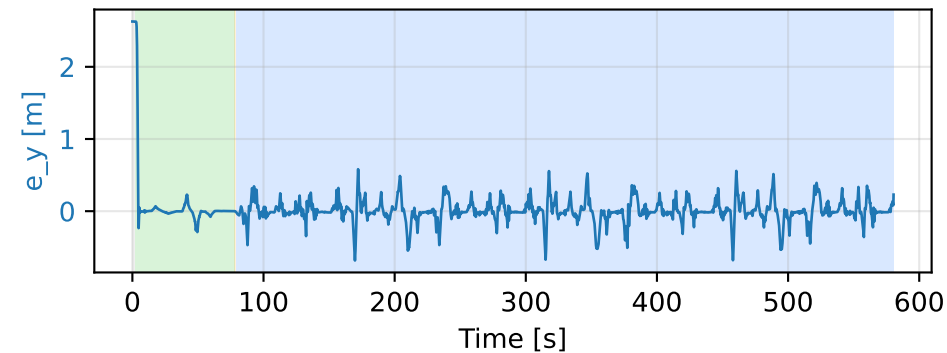
Baseline-NN-MSE
