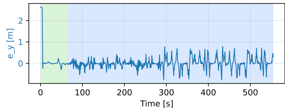
Baseline-NN-MSE
