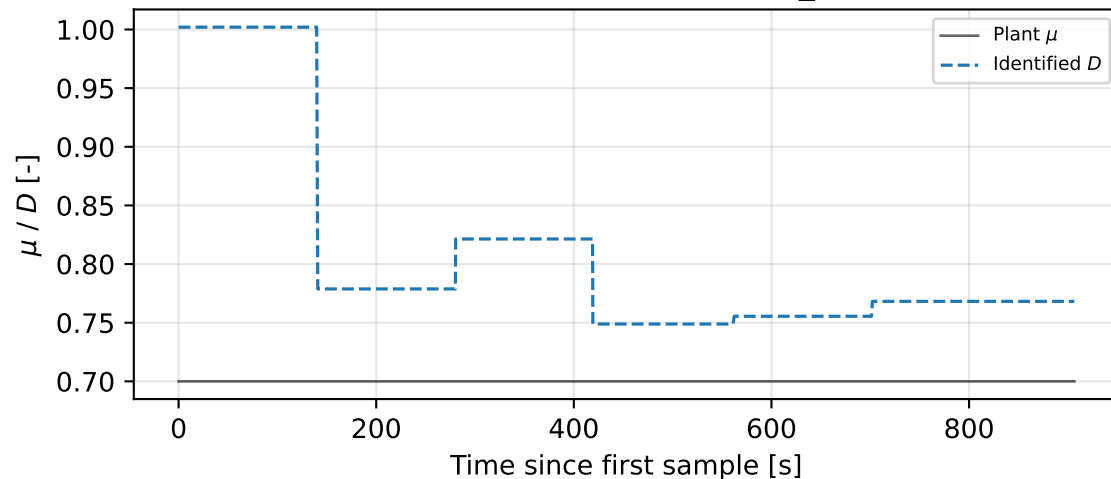
Baseline-NN-MSE - rear_mu
