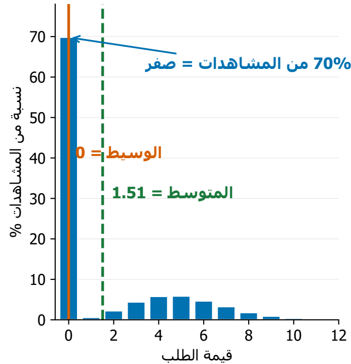
(أ) شكل الطلب المتقطع (D8)
