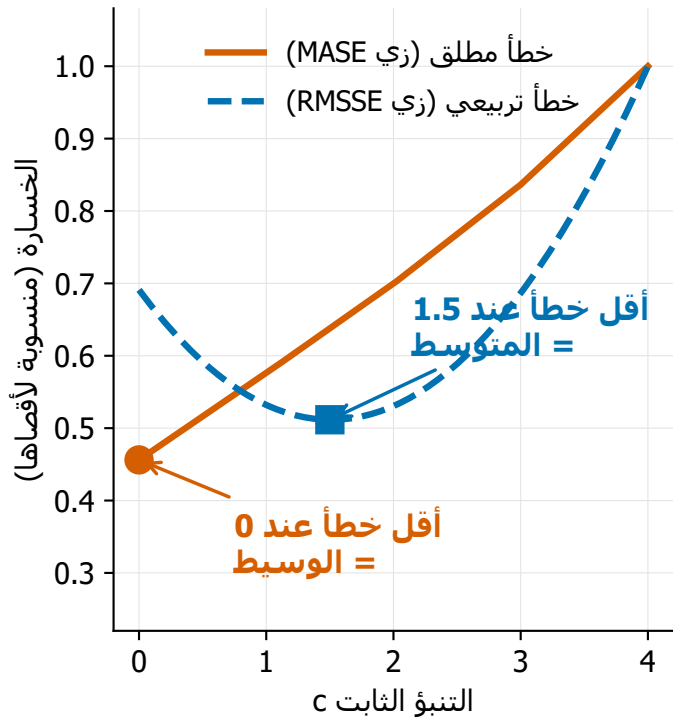
(ب) البرهان: المقياسين عايزين تنبؤ مختلف
