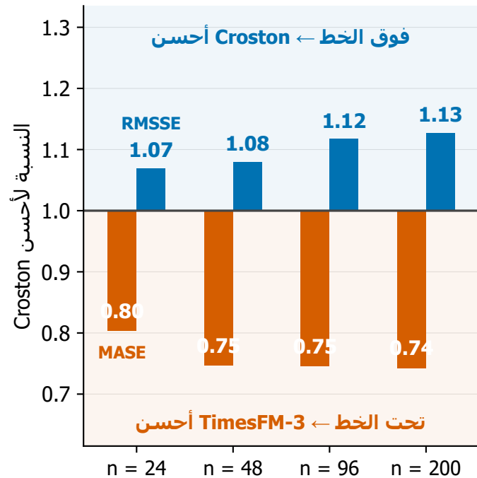
(ج) نفس التنبؤات — والمقياس هو اللي بيحدد الفايز
