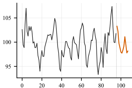
D5: ETS(A,A,A)
