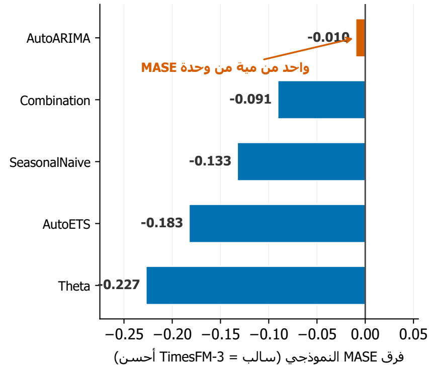
(أ) الفرق معنوي — بس قد إيه؟ (MASE النموذجي \approx 1.05 )
