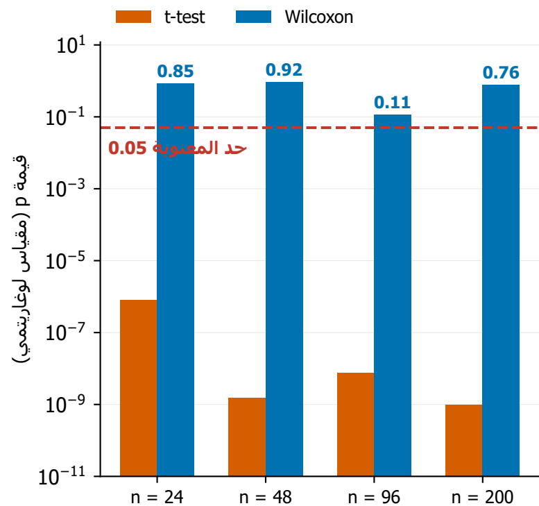
(ج) نفس البيانات — نتيجتين مختلفتين
