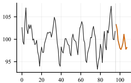
D5: ETS(A,A,A)
