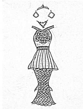
(Mermaid)
