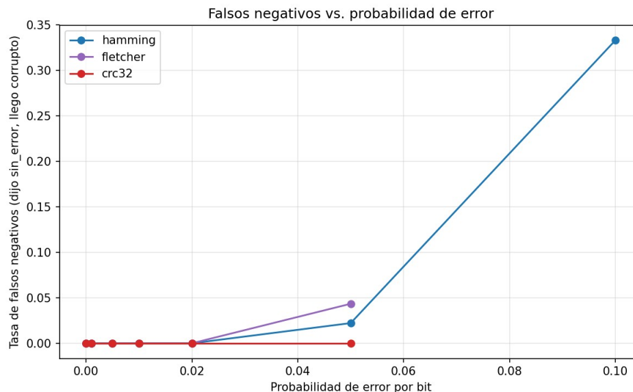
Figura 3. Falsos negativos frente a la probabilidad de error.
