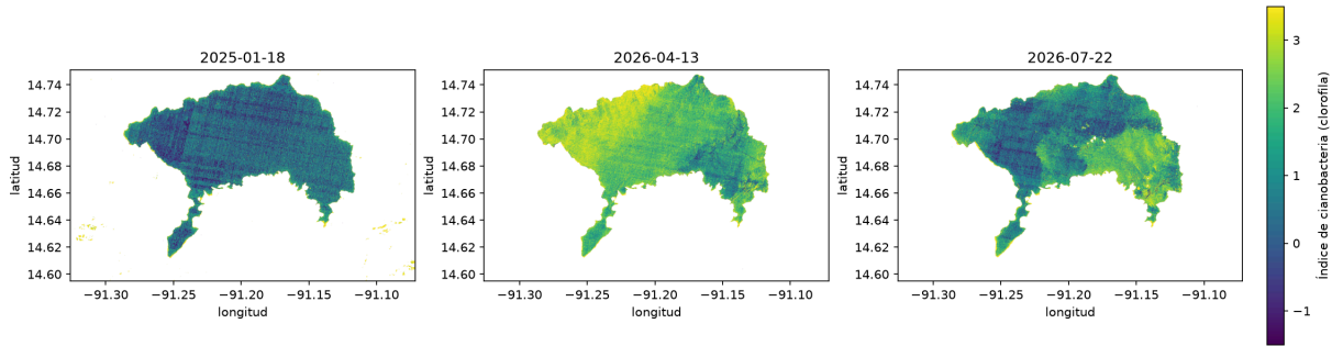
Lago de Atitlán — comparación entre fechas (misma escala)
