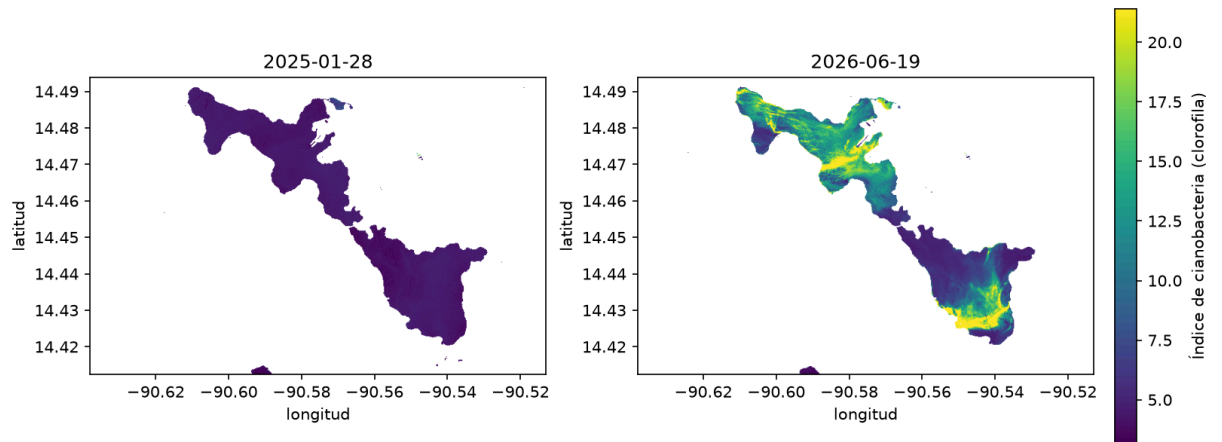
Lago de Amatitlán — comparación entre fechas (misma escala)
