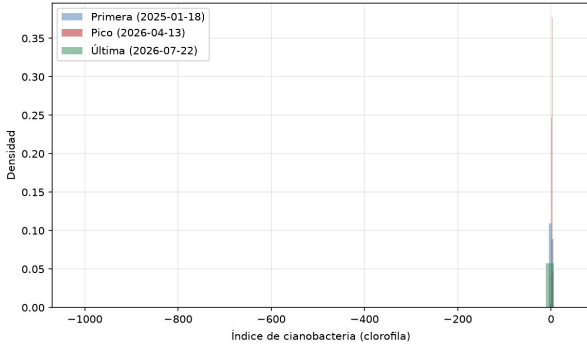
Lago de Atitlán — distribución de cianobacteria en 3 fechas
