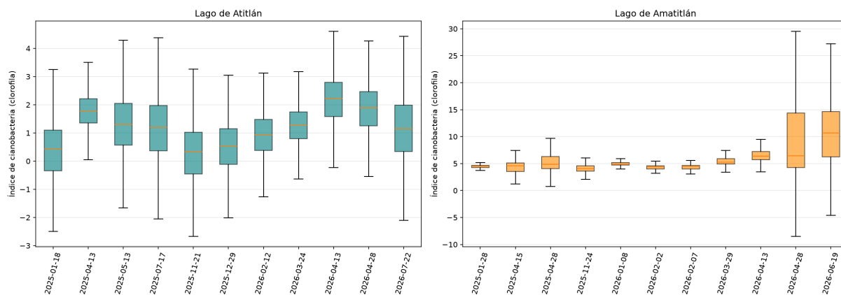
Distribución de cianobacteria por fecha (boxplots, sin outliers)
