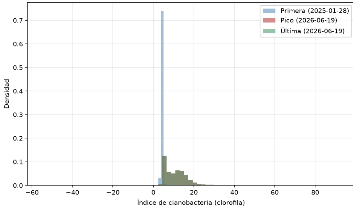
Lago de Amatitlán — distribución de cianobacteria en 3 fechas
