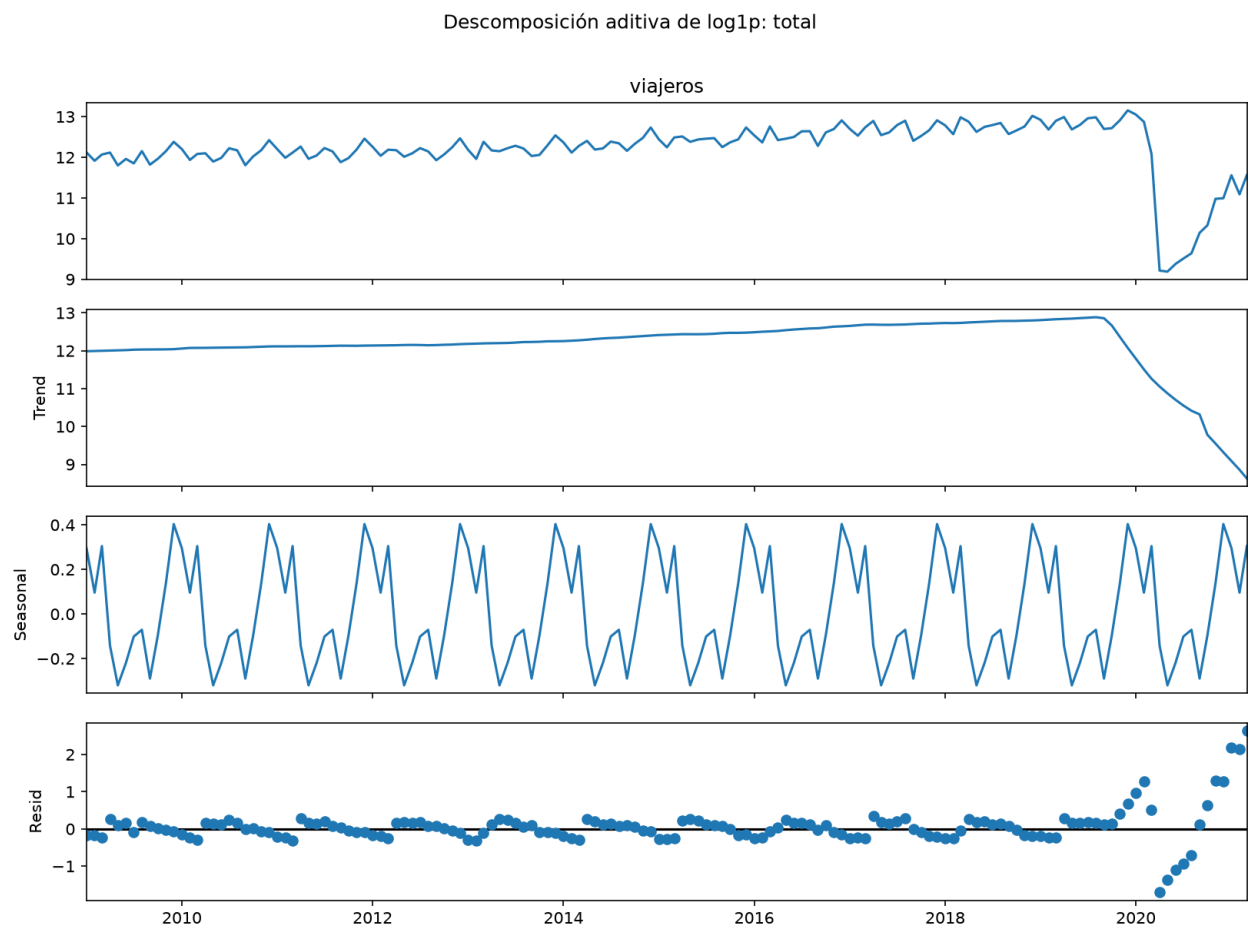
Figure 9: Descomposición de la serie total
