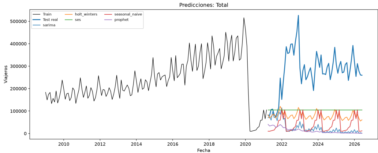
Figure 26: Predicción sobre el conjunto de prueba, total
