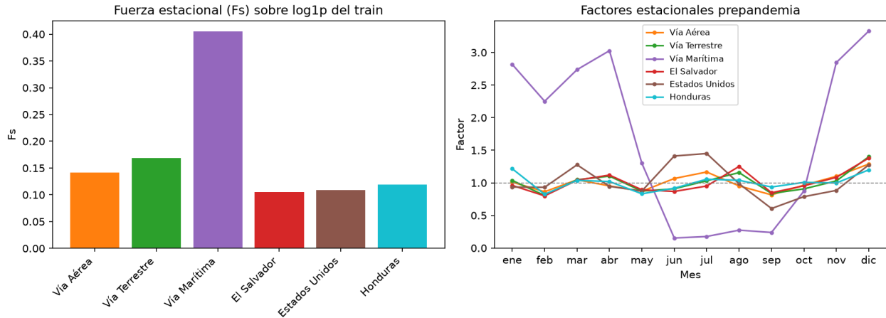
Figure 33: Fuerza estacional por vía de ingreso
