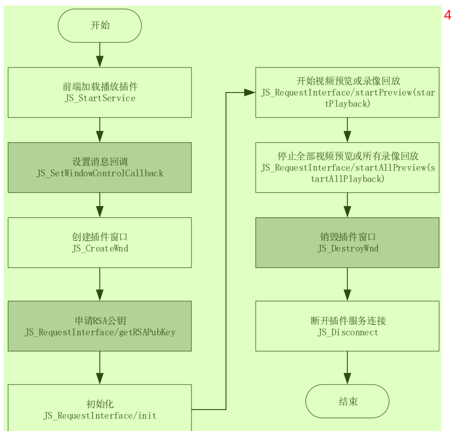
图 4.1-1 VideoWebPlugin 基本对接流程图 5
