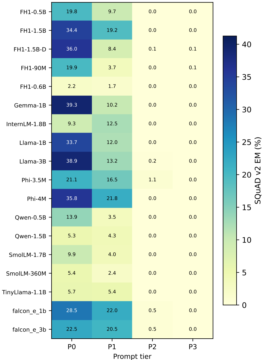
SQuAD v2: Per-Model SQuAD v2 EM (%) (averaged over all edge settings)
