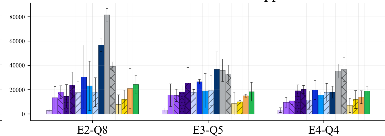
CPU-backed llama.cpp
