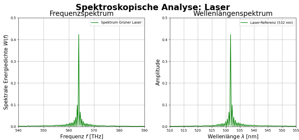
Abbildung 6: Ausschnitt des Laserspektrums in Abhängigkeit der Wellenlänge
