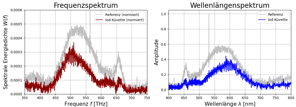
Abbildung 9: Das gemessene Iod-Spektrum in Abhängigkeit von Frequenz und Wellenlänge dargestellt und verglichen mit dem Referenzspektrum der Weißlichtquelle gemessen durch eine leere Küvette
