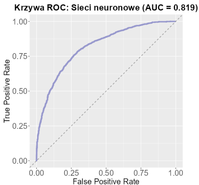
Fig. 20. Wykres krzywej ROC dla metody sieci neuronowych.
