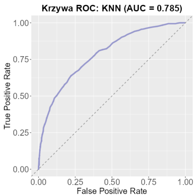
Fig. 24. Wykres krzywej ROC dla metody KNN.
