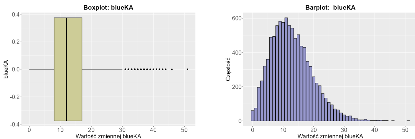
Fig. 13. Boxplot oraz barplot dla zmiennej blueKA .
