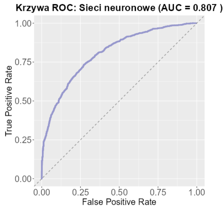
Fig. 20. Wykres krzywej ROC dla metody sieci neuronowych.
