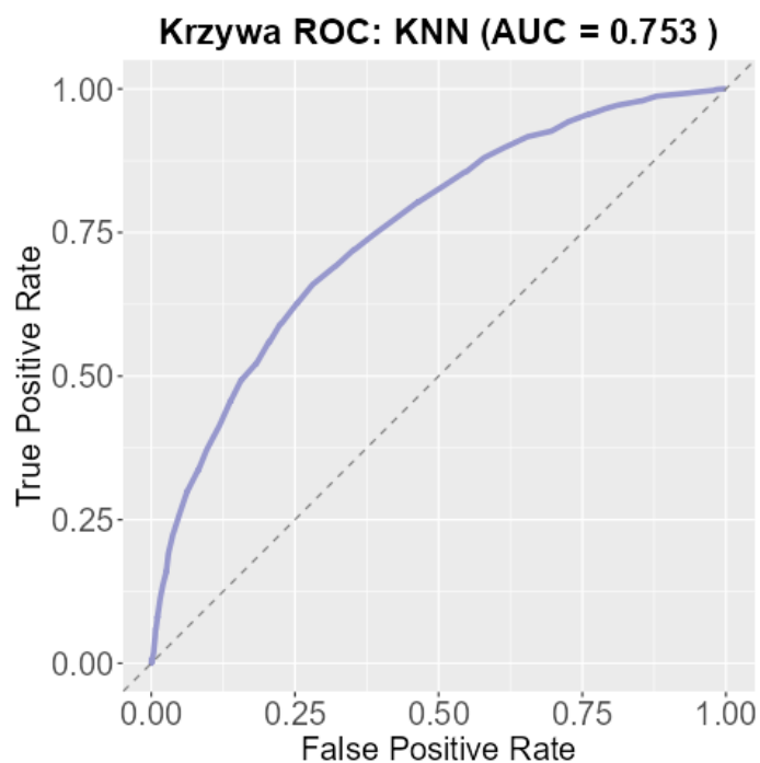
Fig. 24. Wykres krzywej ROC dla metody KNN.
