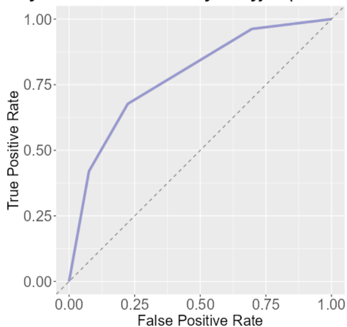
Fig. 22. Wykres krzywej ROC dla metody drzewa klasyfikacyjnego.
