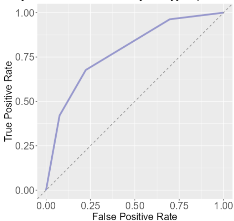
Fig. 22. Wykres krzywej ROC dla metody drzewa klasyfikacyjnego.
