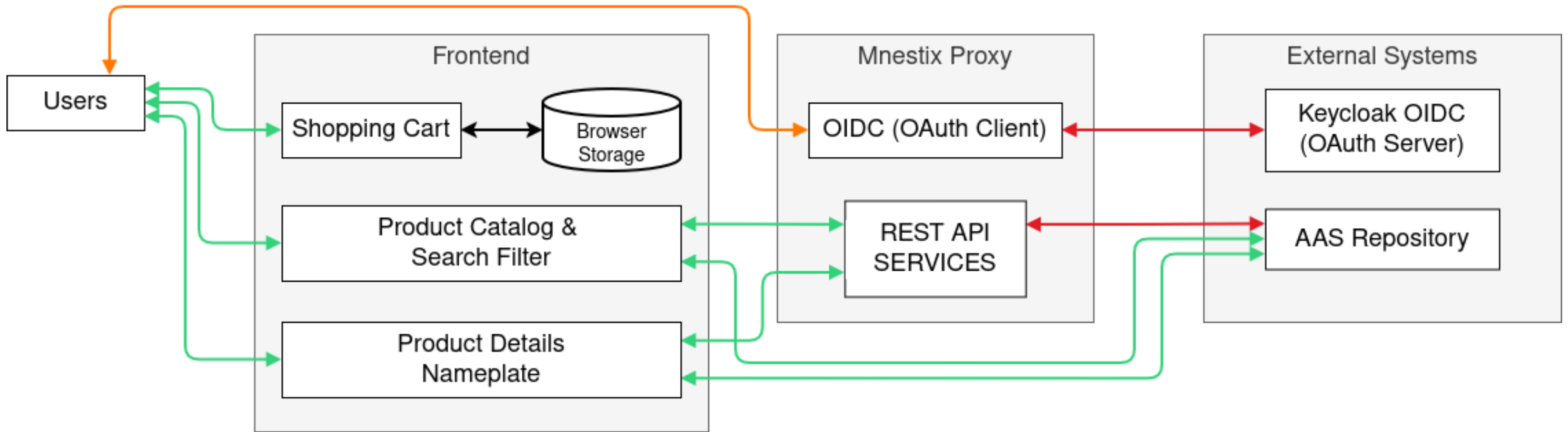
Abbildung: Übersicht über den Software Stack (Quelle: Eigene Herstellung)
