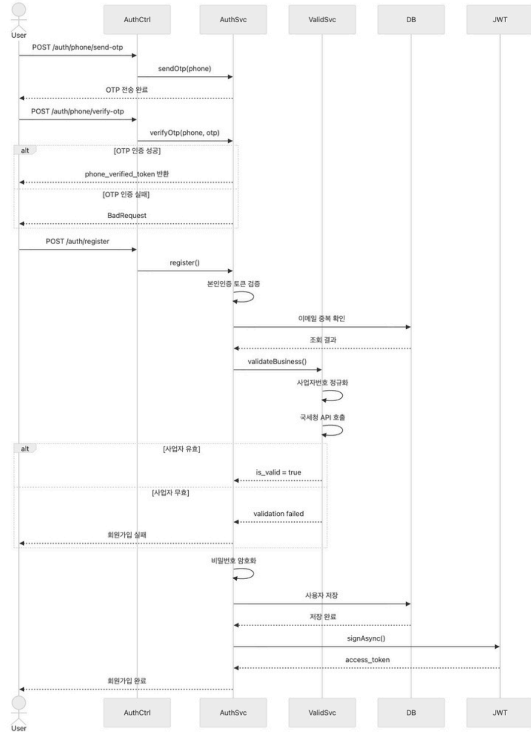
시퀀스 다이어그램
