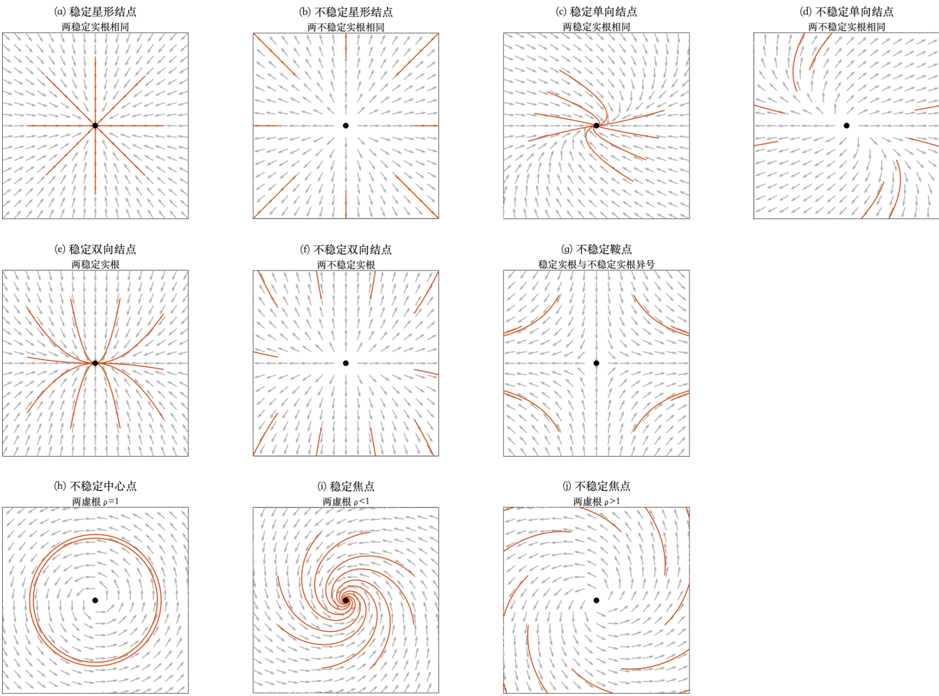
图 1.3: 各种奇点类型汇总图
