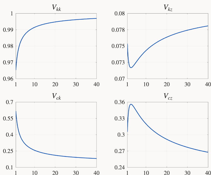
图 10.2: \sigma 上升对迭代系数的影响
