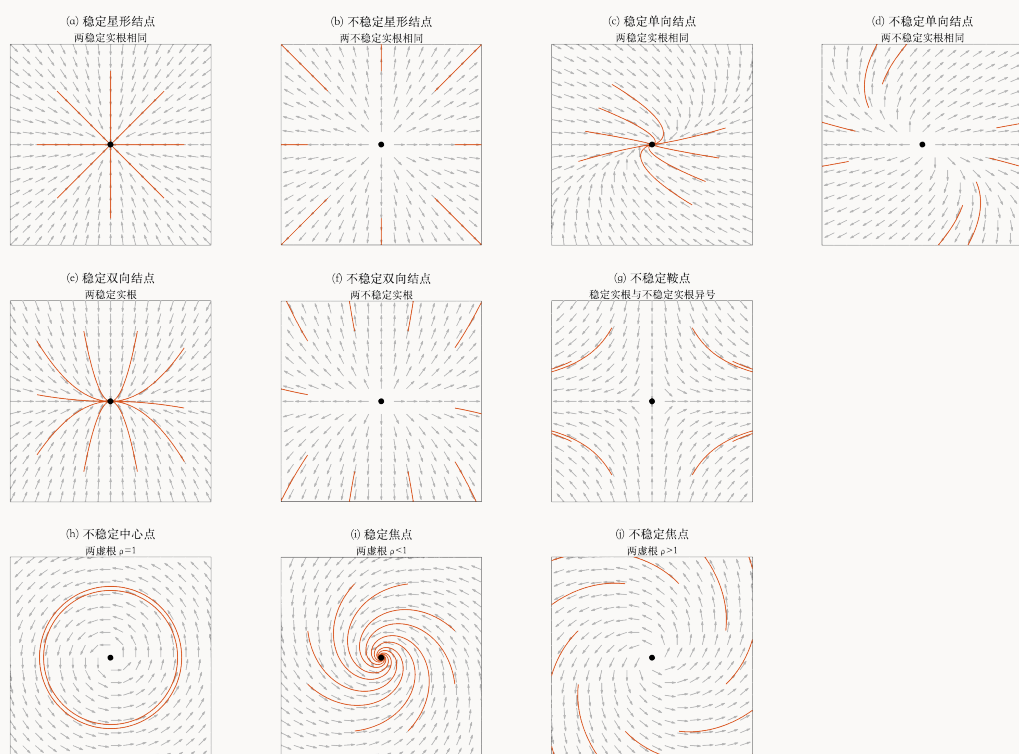
图 7.3：各种奇点类型汇总图
