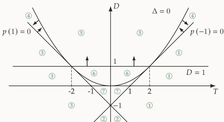
图 7.2: (T, D) 平面中的稳定性分类示意图
