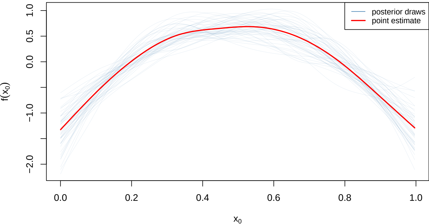
50 posterior draws of s(x_0)
