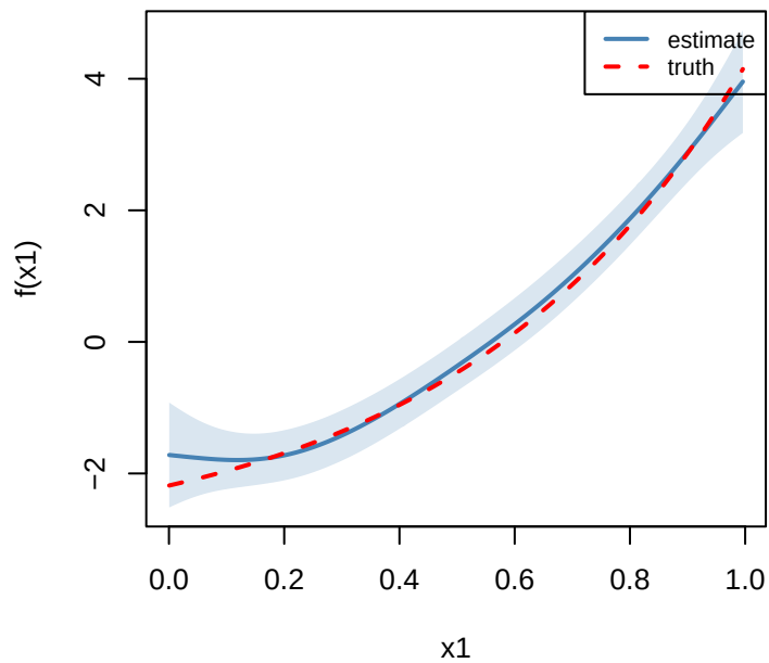
s(x_1)
