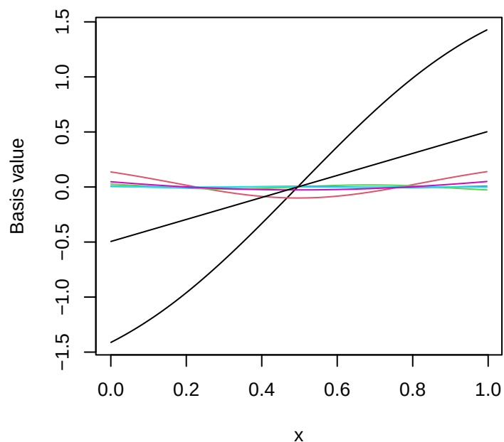
gp basis (k=8)
