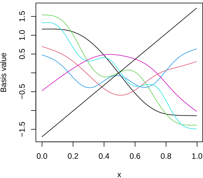
tp basis (k=8)
