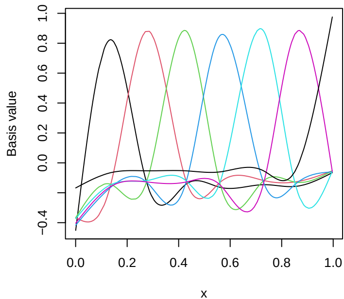
cr basis (k=8)
