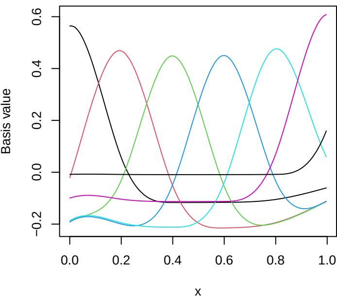
ps basis (k=8)
