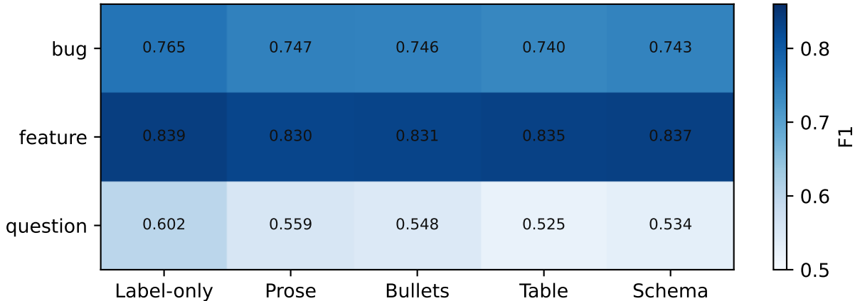
Class-wise F1
