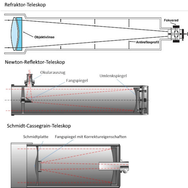
Abbildung 2 – Abbildung der Strahlungsverläufe bei Refraktor-, Newton-Reflektor- und Schmidt-Cassegrain-Teleskopen. Quellen: [22], [23], [24]
