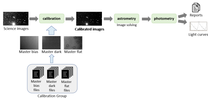
Abbildung 4 – Abbildung eines beispielhaften Stacking-Workflows. Quelle: [57]
