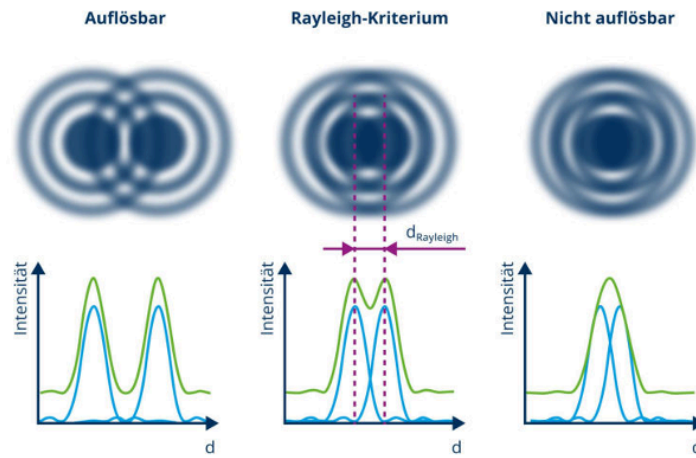
Abbildung 3 – Abbildung der Auflösungsgrenze gemäß dem Rayleigh-Kriteriums mit Intensität der Einzelpunkte. Quelle: [27]
