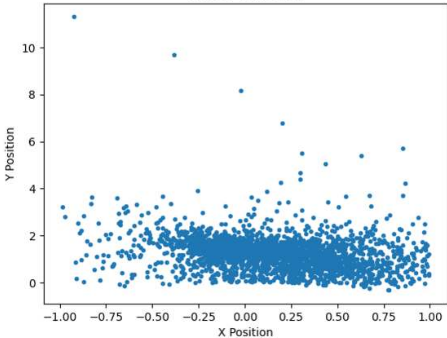
Lander Trajectory
