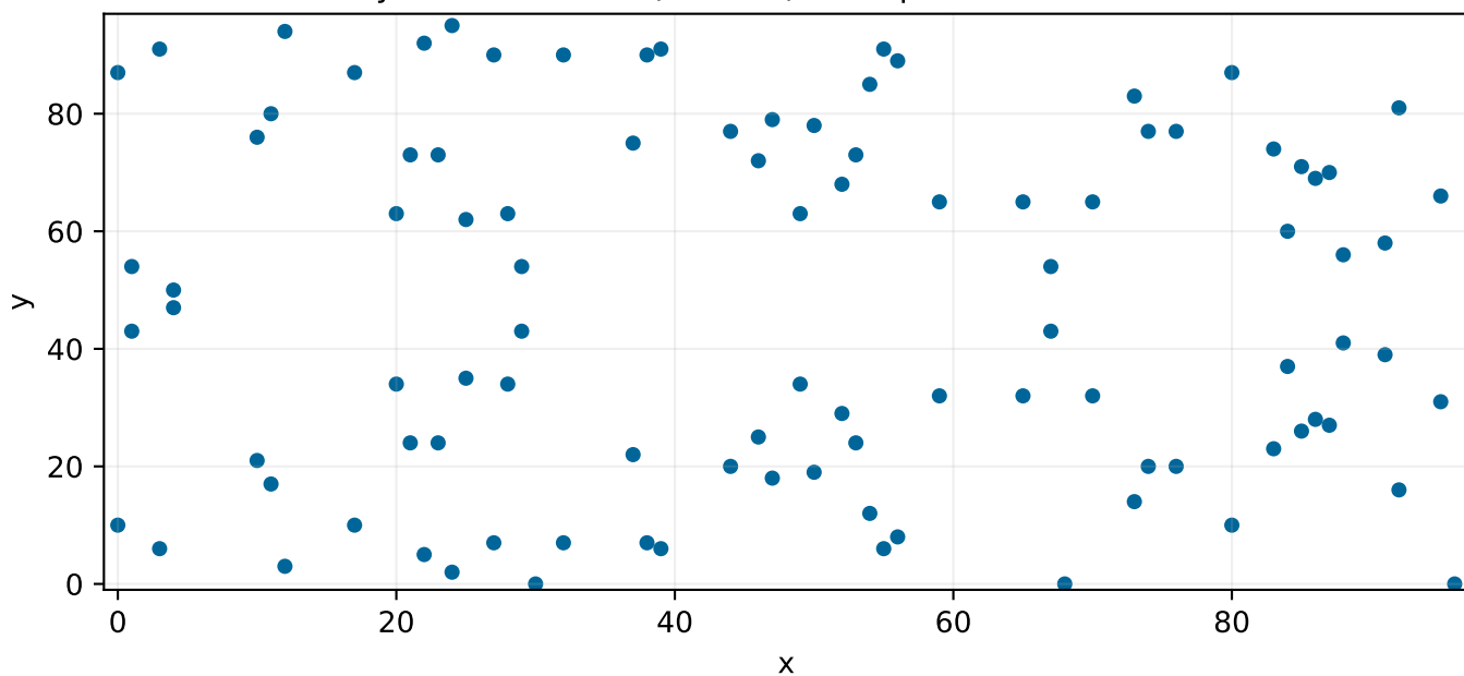
y^2 = x^3 + 2x + 3 \pmod{97} \cdot 100 puntos con infinito
