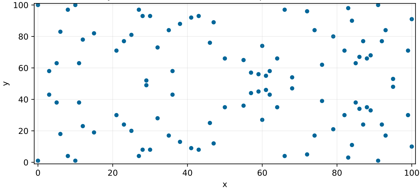
y^2 = x^3 + 1x + 1 \pmod{101} \cdot 105 puntos con infinito
