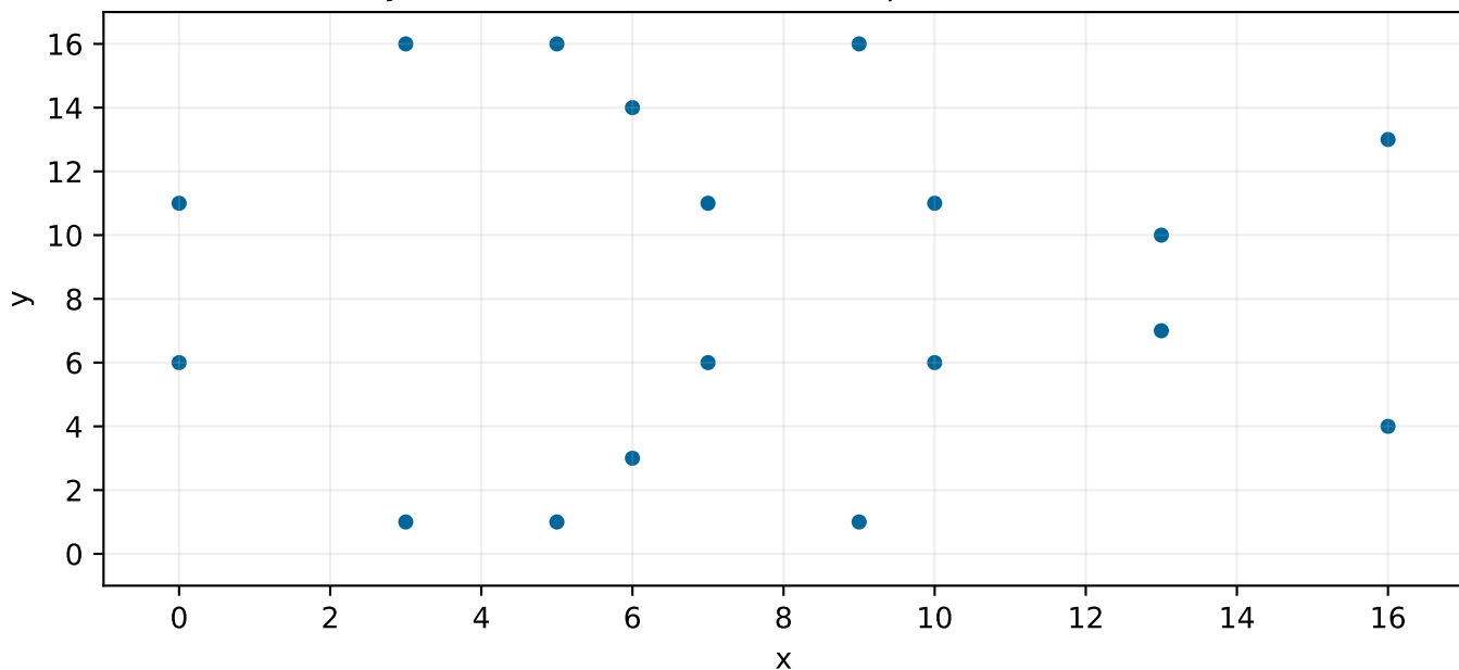
y^2 = x^3 + 2x + 2 \pmod{17} \cdot 19 puntos con infinito
