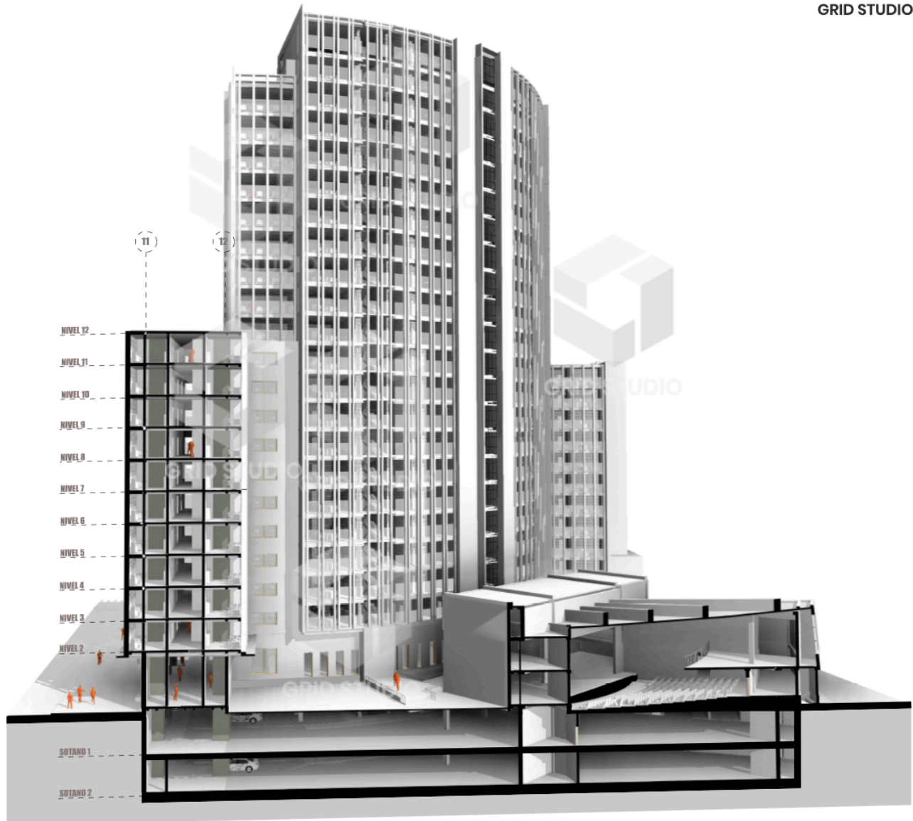
ELEVACIÓN JR. APURIMAC- CORTE FUGADO
