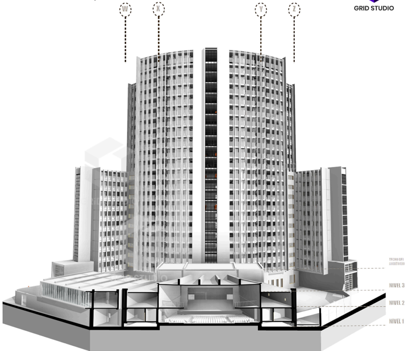
ELEVACIÓN POSTERIOR - CORTE FUGADO
