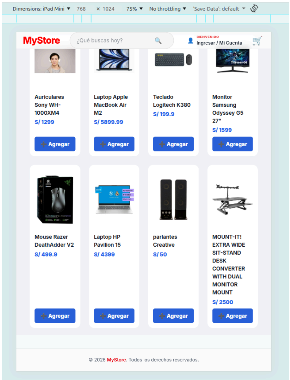
Figura 21 - Responsive en iPad Mini
