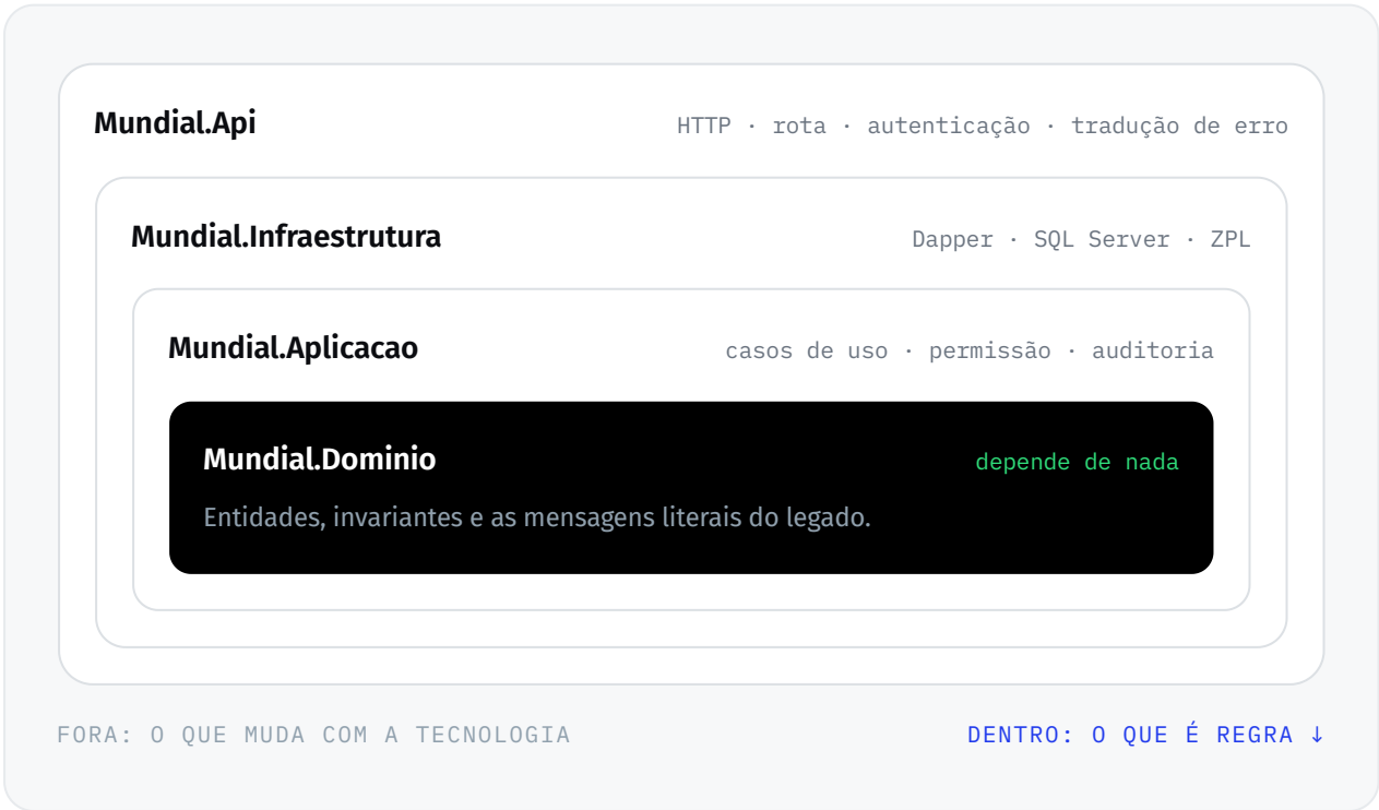
Diagrama 2 — Ports & adapters: a dependência aponta sempre para dentro, e o domínio não referencia nada.
