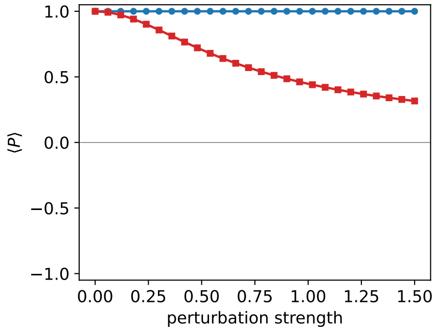
Fermion parity
