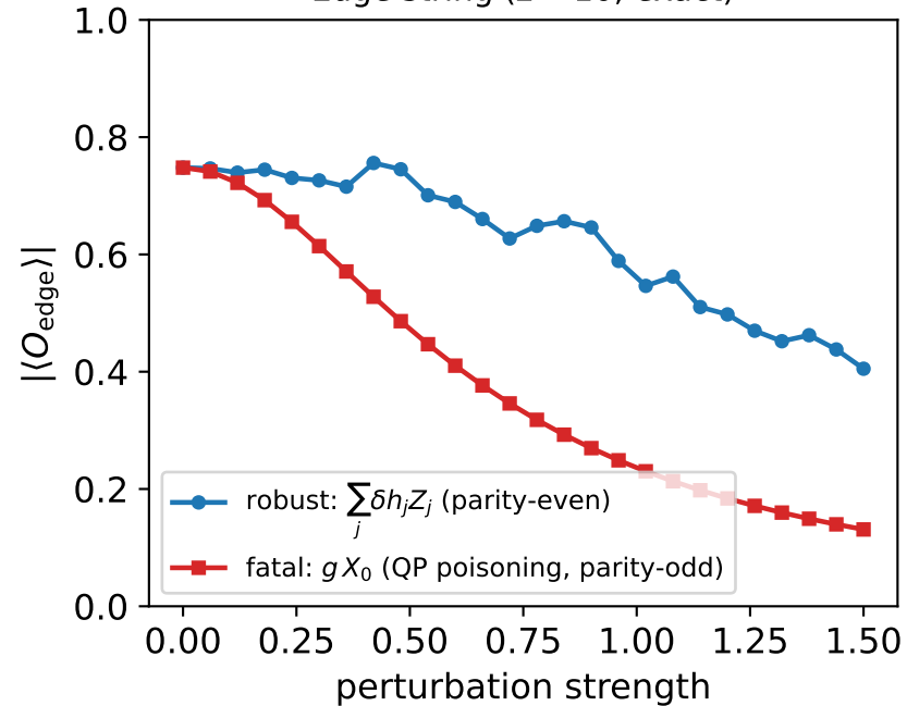
Edge string ( L = 10 , exact)
