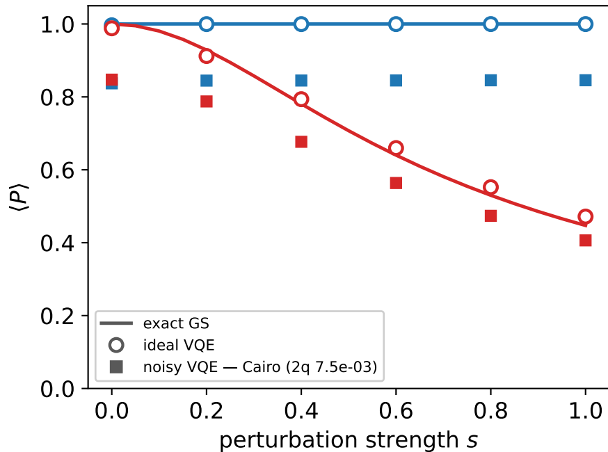
Fermion parity
