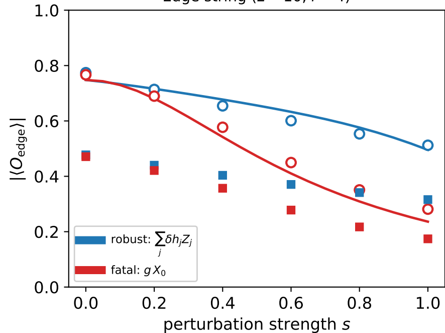
Edge string ( L = 10, r = 4 )
