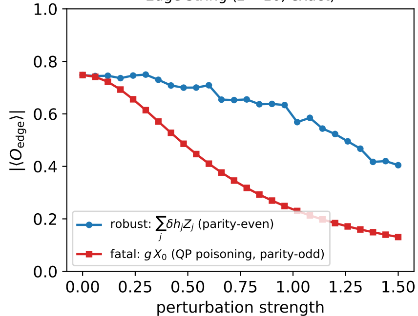
Edge string ( L = 10 , exact)
