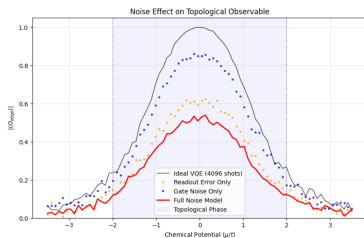
(b) ReadoutError:0.11, GateError:0.7
