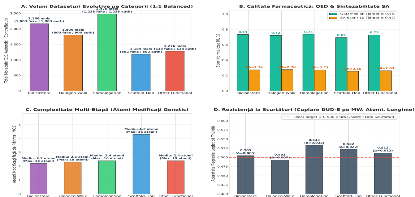
Evaluarea Dataseturilor Evolutive Condiționate pe Categoriile (NSGA-II Anti-Shortcut)
