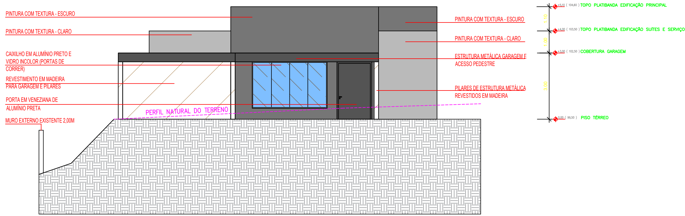
04 ELEVACÃO 02 ESCALA 1/100
